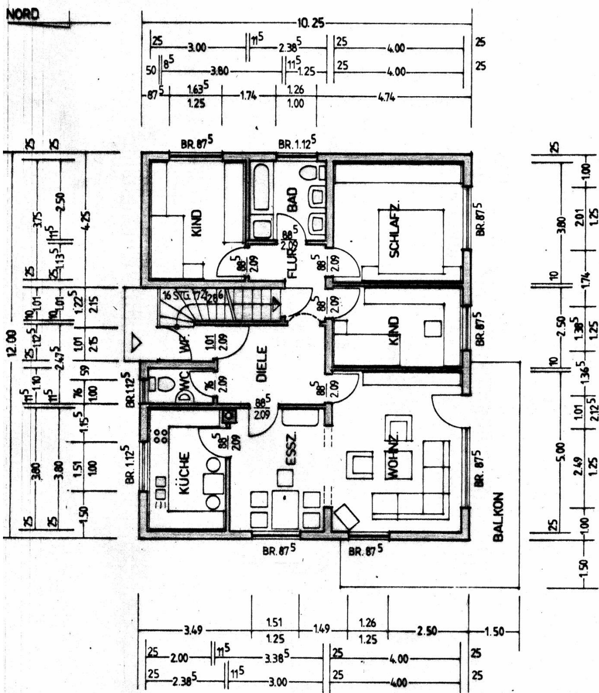
ERDGESCHOSS M. 1:100
